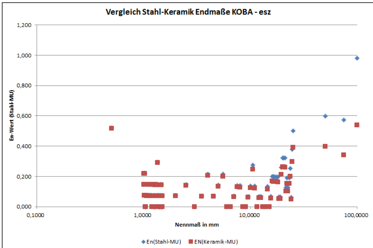
En-Auswertung vom 4.12.2012 zwischen KOBA und esz bei Vergleich gegen den Bezugsnormalendmaßkasten aus Stahl.
